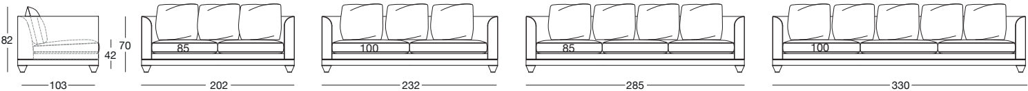
Terminali Sx / End unit L.H. / Боковые секции Л
