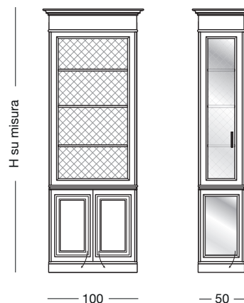
Moduli speciali boiserie / boiserie special panels Специальные модули буазери
