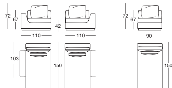
Dormeuse / Dormeuse / Дормез
