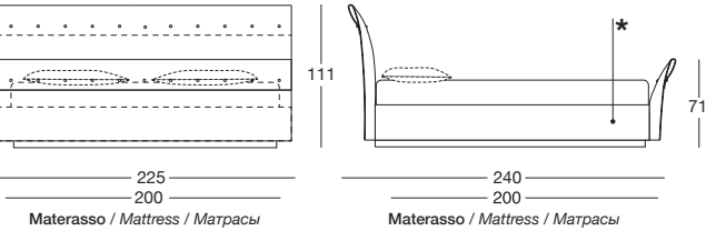
Giroletto con pediera a bottoni / bedframe with footrest with buttons Каркас кровати с изножьем с пуговицами
