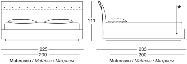
Giroletto con pediera imbottita 10 cm / bedframe with upholstered 10 cm footrest Каркас кровати с мягким изножьем 10 см
