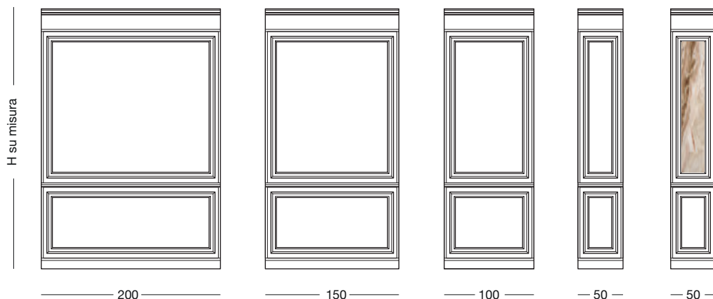
Moduli boiserie / boiserie panels Модули буазери
