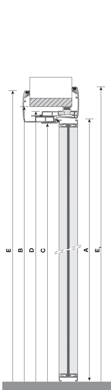
Porta standard - stipite TONDO Standard door - ROUND jamb Стандартная дверь - КРУГЛЫЙ косяк
