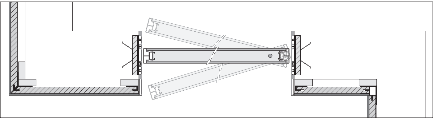
Porta con apertura a bilico bidirezionale e boiserie Two-way bi-directional door with boiserie | Маятниковая дверь с открытием в двух направлениях с буазери
