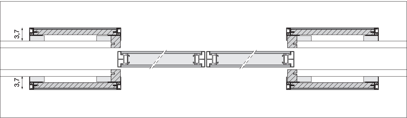
Scorrevole a scomparsa a due ante con boiserie a filo da due lati Double pocket door with flush boiserie on both sides | Двустворчатая раздвижная дверь с уходом в стену с буазери заподлицо с 2 сторон
