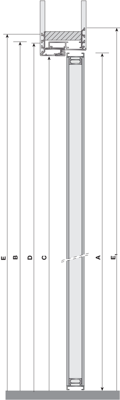
Porta doppia - stipite FILOMURO IANUS Double swing door - FILOMURO IANUS jamb Двойная дверь - Косяк FILOMURO IANUS
