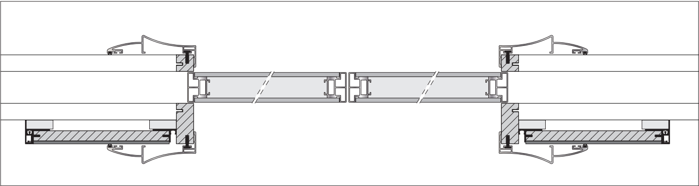
Scorrevole a scomparsa 2 ante con boiserie 1 lato Double pocket doors with boiserie on one side | 2-створчатая раздвижная дверь с уходом в стену с буазери с 1 стороны
