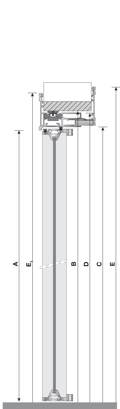
Porta standard - stipite WAVE Standard door - WAVE jamb Стандартная дверь - Косяк WAVE
