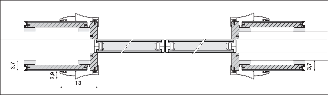
Scorrevole a scomparsa a due ante con boiserie da due lati Double pocket door with boiserie on both sides | Двустворчатая раздвижная дверь с уходом в стену с буазери с 2 сторон
