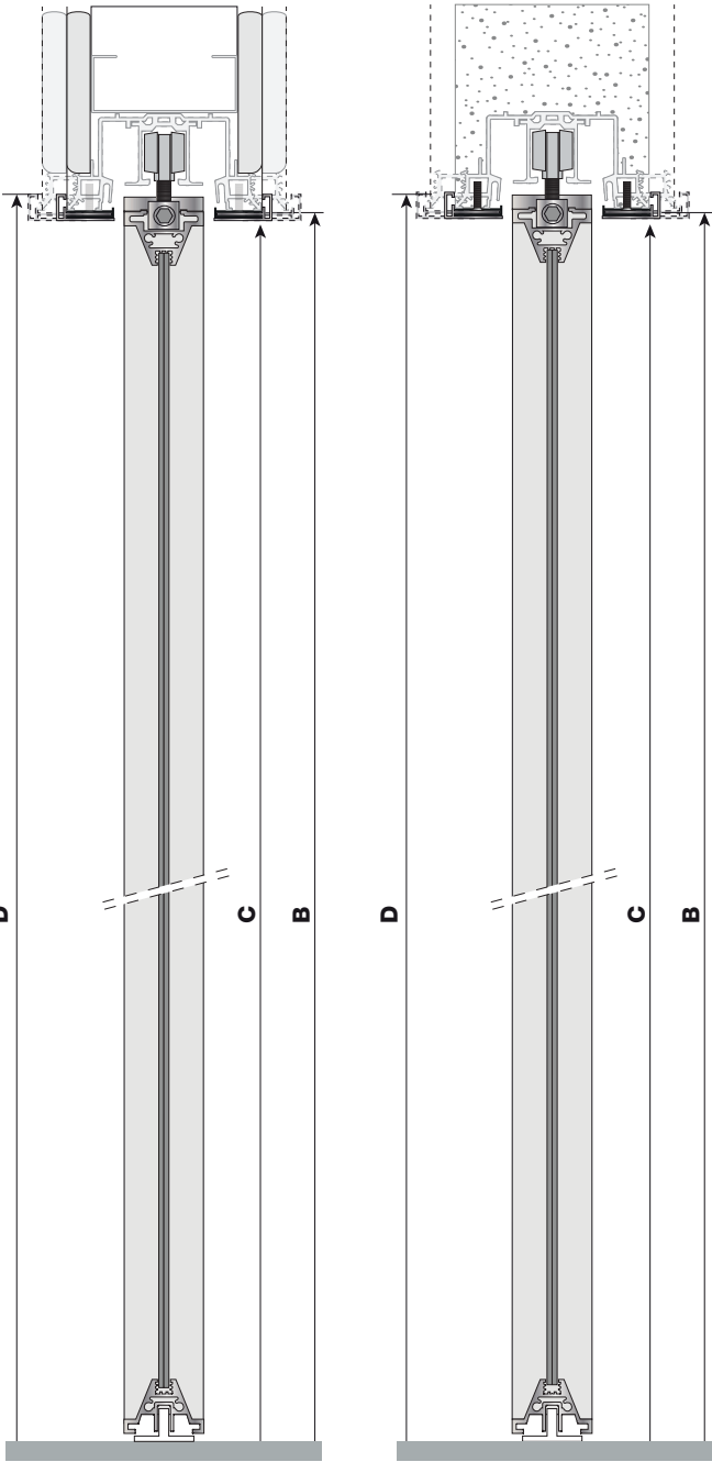
Stipite FREE - cartongesso FREE jamb - plasterboard Косяк FREE - гипсокартон Stipite FREE - intonaco FREE jamb - plaster Косяк FREE - штукатурка
