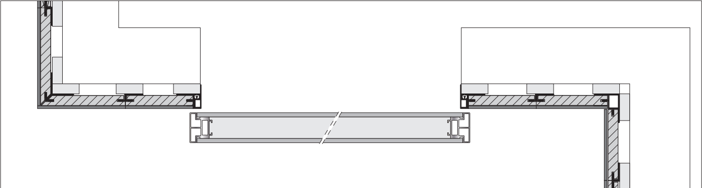
Pannello scorrevole e boiserie Sliding panel with boiserie | Раздвижная панель с буазери
