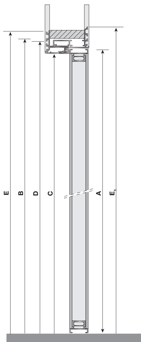
Porta standard - stipite FILOMURO IANUS Standard door - FILOMURO IANUS jamb Стандартная дверь - Косяк FILOMURO IANUS
