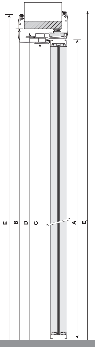
Porta doppia - stipite TONDO Double swing door - ROUND jamb Двойная дверь - КРУГЛЫЙ косяк
