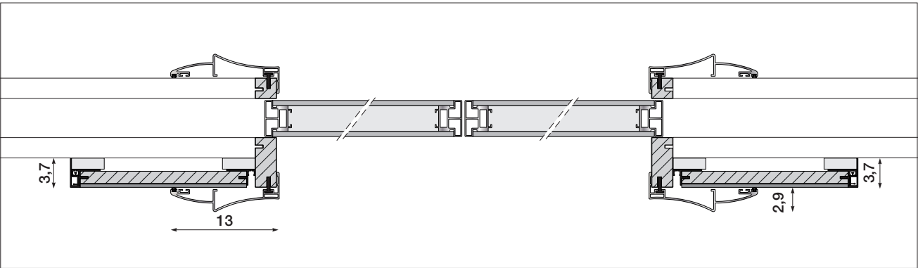
Scorrevole a scomparsa a due ante con boiserie da un lato Double pocket doors with boiserie on one side | Двустворчатая раздвижная дверь с уходом в стену с буазери с 1 стороны
