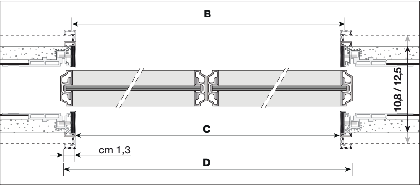
Stipite FREE - cartongesso FREE jamb - plasterboard Косяк FREE - гипсокартон Stipite FREE - intonaco FREE jamb - plaster Косяк FREE - штукатурка
