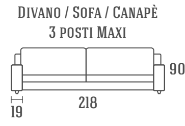
DIVANO / SOFA / CANAPÈ 3 POSTI
